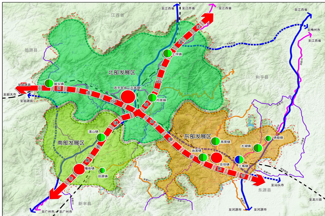
“一廊两轴两心多组团”发展格局图
