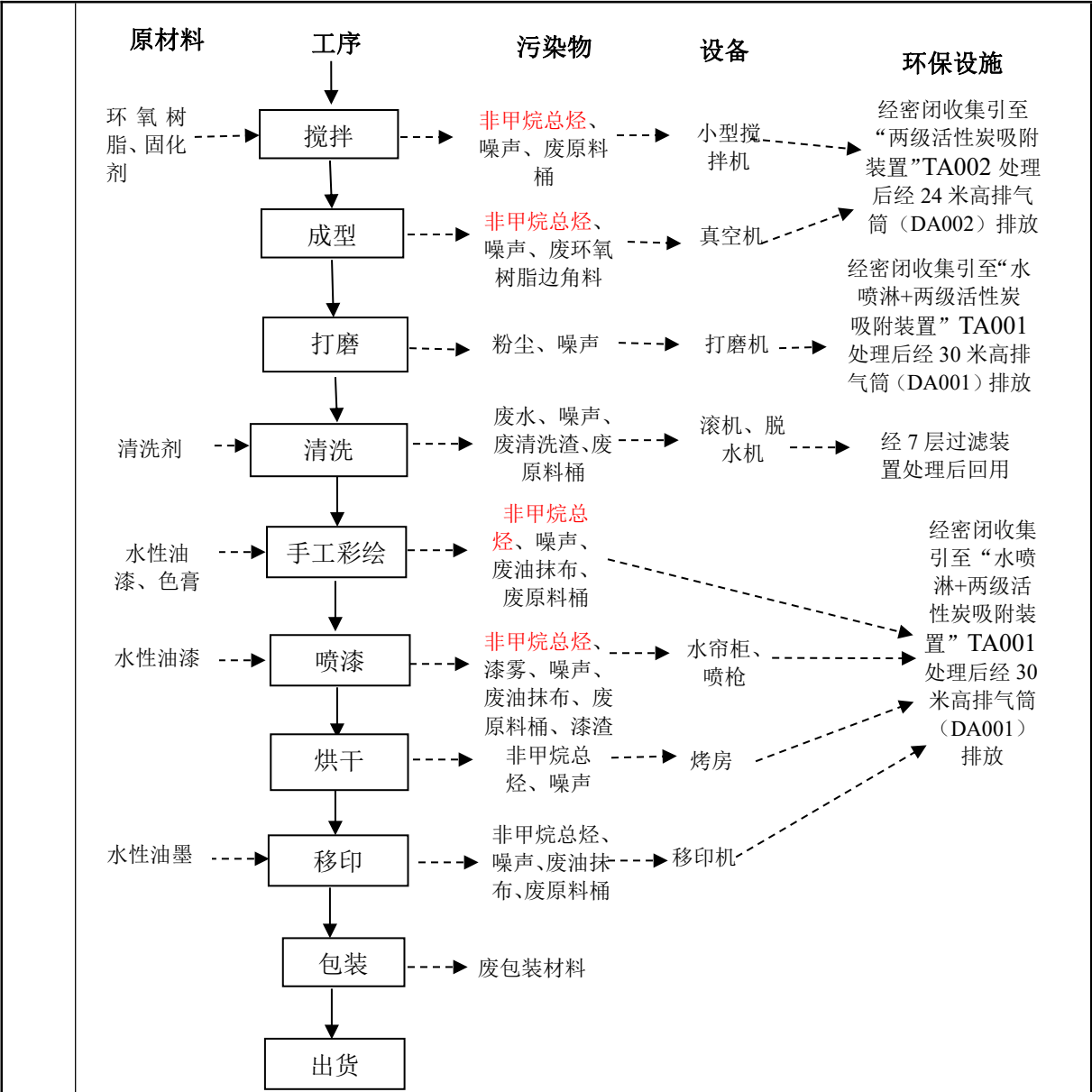
图 2-2 运营期环氧树脂制品生产工艺流程及主要产污环节图
